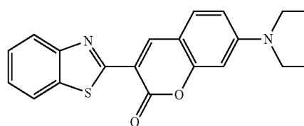
Coumarin 6
