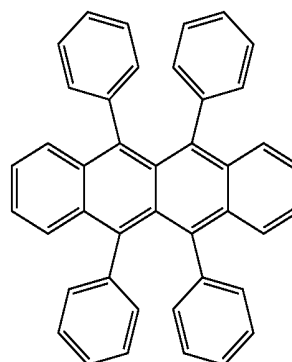
Rubrene
